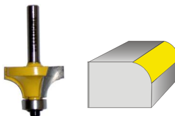
FRESA PARA REDONDEAR ESQUINAS CON RODAMIENTO GUIA DE 1/2"
