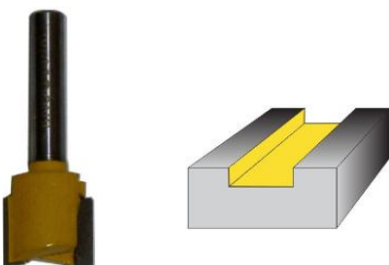
FRESA PARA MORTAJAR ESPECIAL PARA HACER CAJAS
