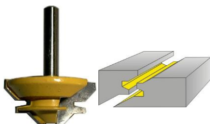
FRESA PARA UNION O EMPALME REF: 22620
