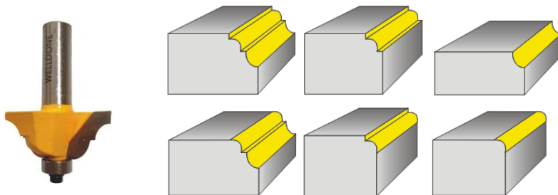
FRESA DE CORTES CLASICOS REF: 22751 - 22852
