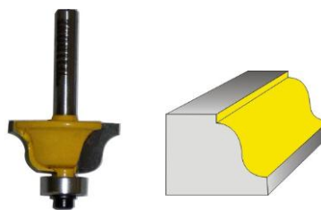
FRESA PARA MOLDURA TIPO PECHO PA- LOMA
