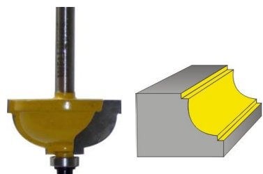
FRESA CONCAVA PARA BORDEAR REF: 22840 - 22842 - 22858 - 22589
