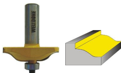
FRESA PARA REALZAR PANELES REF: 22837 - 22839 - 22854 - 22856
