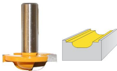
FRESA PARA HACER CAJAS DE CAZUELAS REF: 22829
