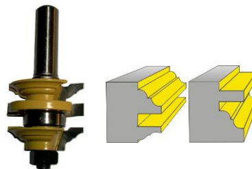
FRESA PARA ENCAJE Y EMPALME REF: 22857
