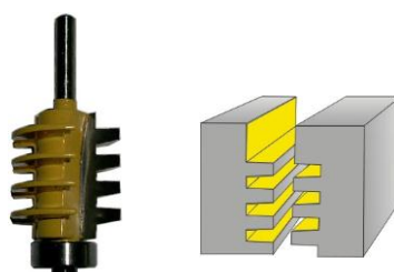
FRESA PARA UNION O EMPALME REF: 22621
