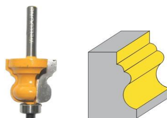
FRESA PARA PERFILAR
