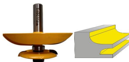
FRESA EN CONJUNTO DE DOS CUCHILLAS REF: 22833
