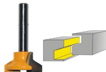
FRESA PARA HACER CORREDERA CAJON REF: 22349 - 22350
