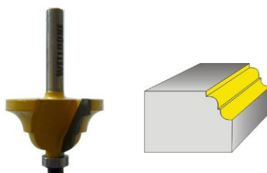
FRESA CORTE CLASICO REF: 22752 - 22753 - 22755 - 22850
