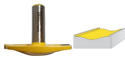
FRESA CORTE CLASICO REF: 23737 - 23838
