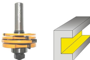
FRESA PARA RANURAR DE DISCOS INTER- CAMBIABLES REF: 22670
