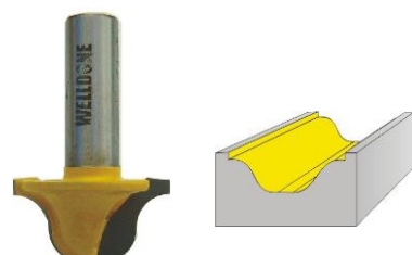
FRESA DE CORTE TIPO PECHO PALOMA REF: 22788 - 22789 - 22864 - 22866
