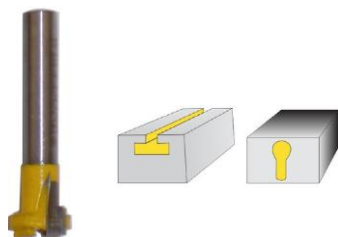
FRESA PARA HACER RANURAS DE EXHIBIDORES
