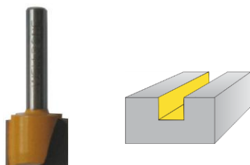
FRESA PARA CORTE RECTO CON CUCHILLA INFERIOR PARA CORTE EN EL FONDO
