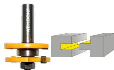
FRESA PARA UNION O EMPALME REF: 22775 - 22877
