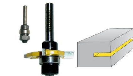
DISCO PARA RANURAR CON 3 PUNTAS ARBOL DE 1/2"
